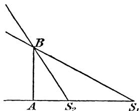
FIG. 72.—The Gnomon.
